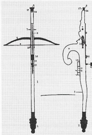
Doorsnede St. Jansboog of balansboog
