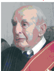
Johan van Schijndel
