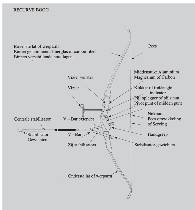
Schematische voorstelling van de handbogen. Recurvehandboog (l) en compoundhandboog
